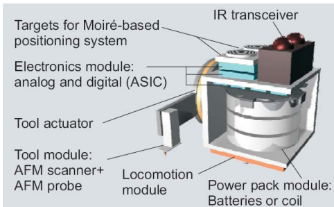
Fig. 1. MiCRoN robot
